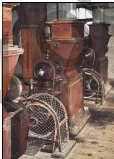
Abb. 4.12.21: Walzenstühle.
