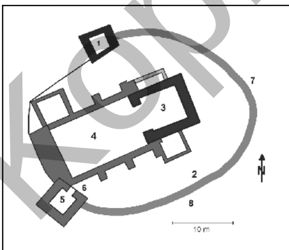
Abb. 4.3.1: Grundriss der heutigen Kirche nach Torke, M. [4.48]. 1 Torgebäude, 2 Ringmauer, 3 Chor, 4 Kirchenschiff, 5 Turm mit Schießscharten, 6 Ringmauer, 7 Halsgraben, 8 Ringgraben.
