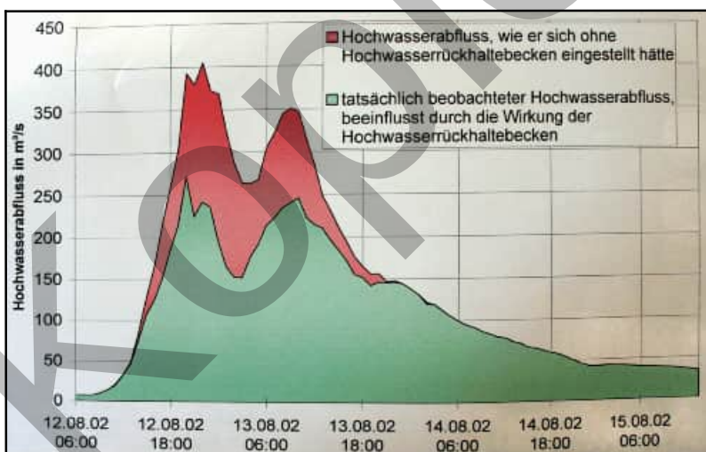
Abb. 4.9.2: Abflussverhältnisse mit und ohne Talsperrensystem bei dem Hochwasser 2002. Abb. nach [4.29].
