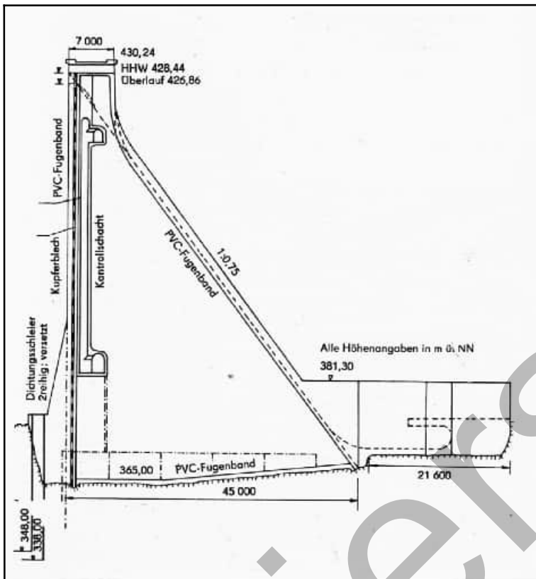
Abb. 4.9.1: Schnitt durch die Staumauer. Abb. nach [4.29].
