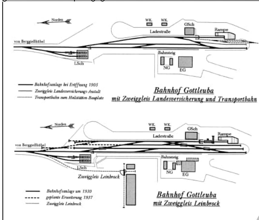
Abb. 4.1.14: Gleisplan Bahnhof Gotttleuba mit dem Anschluss Landesversicherung 1905. EG - Empfangsgebäude, LSch - Lokschuppen, GSch - Güterschuppen, NG - Nebengebäude [4.9].
