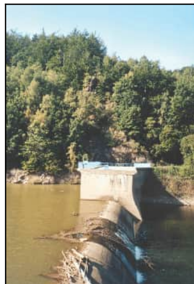
Abb. 4.9.14: Vorsperre 2003.
