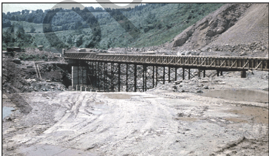
Abb. 4.9.7: Das neue Bett der Gottleuba über der Gründung 1968. Samml. Jürgen Freitag, Oelsen.
