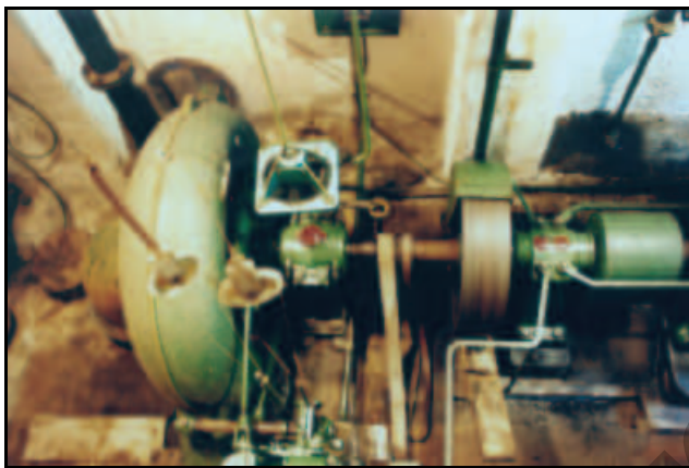
Abb. 9.1.154: Die alte 120 kW-Kleinwasserkraftanlage 2002.
