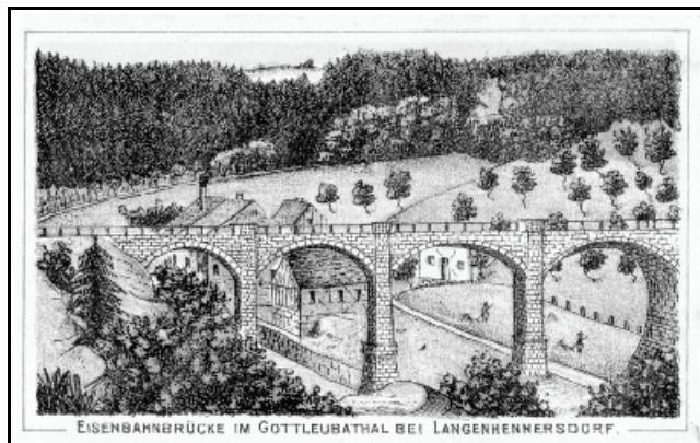
Abb. 9.1.8: Die alte Steinbrücke von 1880 unterhalb des Bahnhofes Langenhennersdorf. Blick flussabwärts.
