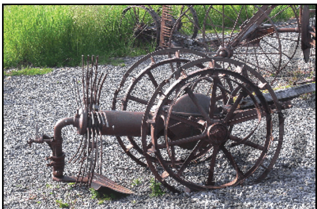
Abb. 1.10.39: Kartoffelroder aus den 1940er Jahren.
