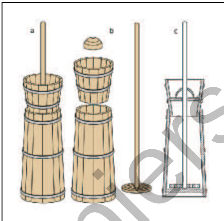
Abb. 1.10.52: Aufbau eines Butterfasses. Quelle: Wikipedia.
