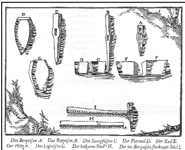
Abb. 1.3.6: Bergeisen. Quelle: Agricola [1.1].
