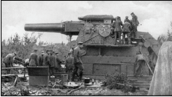
Abb. 1.8.5: Das deutsche Großgeschütz "Dicke Berta" von Krupp an der Front vor Lüttich 1914. Erst mit diesem Geschütz konnten die Forts erobert werden. Foto: Wikipedia
