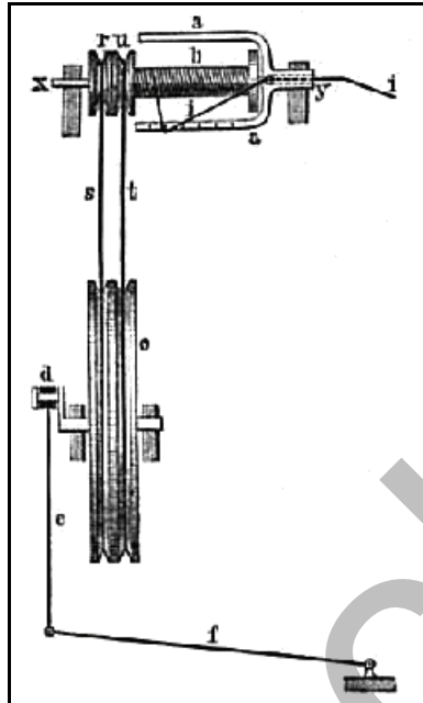
Abb. 1.5.19: Aufbau des Spinnrades. Wikipedia.
