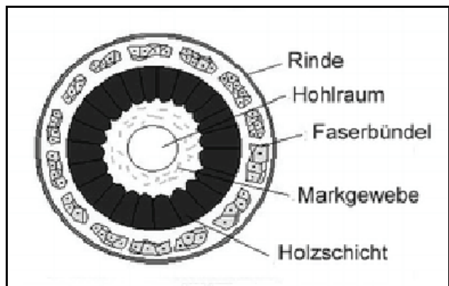
Abb. 1.5.22: Aufbau eines Flachsstengels. Wikipedia.
