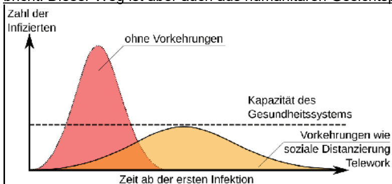
Abb. 1.11.11: Infektionsverlauf ohne und mit Vorkehrungen. Abb. Wikipedia.
