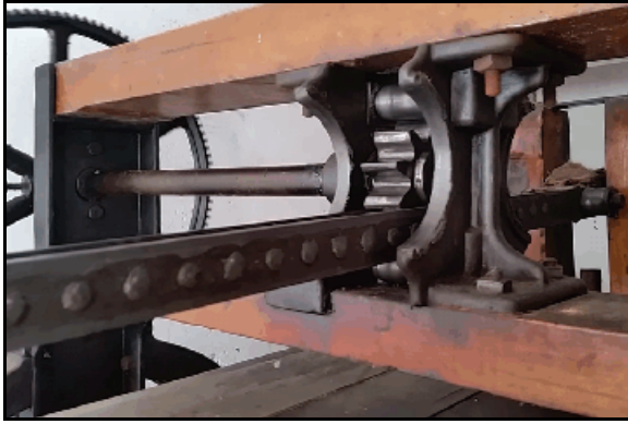
Abb. 1.10.19: Der Kasten Antrieb mit Zahnstange.
