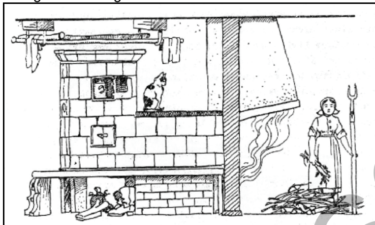
Abb. 1.5.9: Der Altdeutsche Ofen. Nach Lohse.
