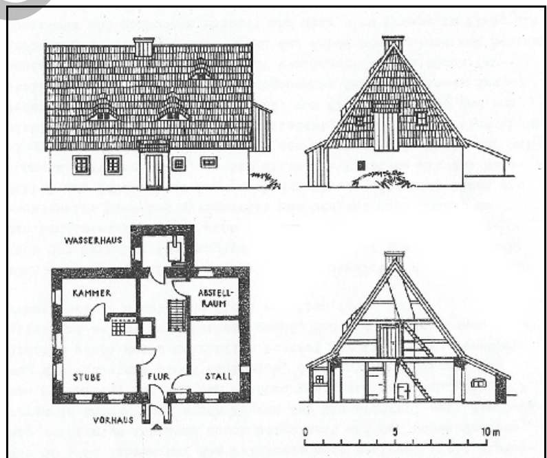
Abb. 1.5.3: Aufbau eines Häuslerwohnhauses (Arbeiterwohnhauses) nach Helbig [1.24] in Neugeorgenfeld von 1732.
