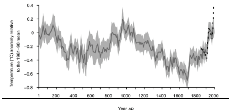
Abb. 1.13.1: Temperaturabweichung von dem Mittelwert in den letzten 2000 Jahren auf der nördlichen Hemisphäre nach Ljungquist 2010 [1.46].
