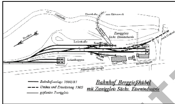
Abb. 5.1.11: Gleisplan Bahnhof Berggießhübel.
