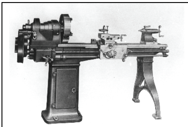
Abb. 5.13.28: Kleine Drehbank der Berggießhübler Werkzeugmaschinenfabrik von 1938. Foto: Samml. Gerold Häbig, Oelsen
