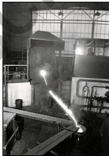
Abb. 5.13.17: Abguss aus dem Elektroofen. Foto: Samml. Frau Streit.
