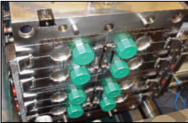
Abb. 5.13.39: Gusswerkzeug. Werksfoto "Bergi-Plast" 2011.
