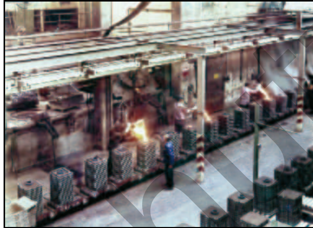
Abb. 5.13.11: Die Gießstraße mit Elektroinduktionsöfen 1974. Foto: Samml. Frau Streit, Bergg.
