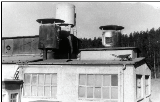
Abb. 5.13.19: Die drei Kupolöfen 1984. Foto Samml. Frau Streit, Bergg.
