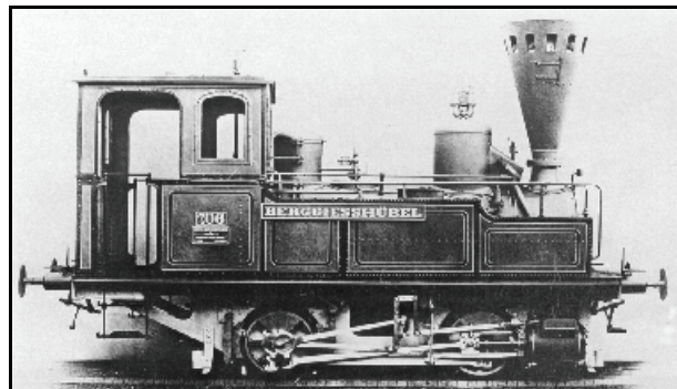
Abb. 5.1.9: Die zweiachsige Tenderlok H.VII T "Berggießhübel" von der Gießerei Hartmann, Chemnitz.
