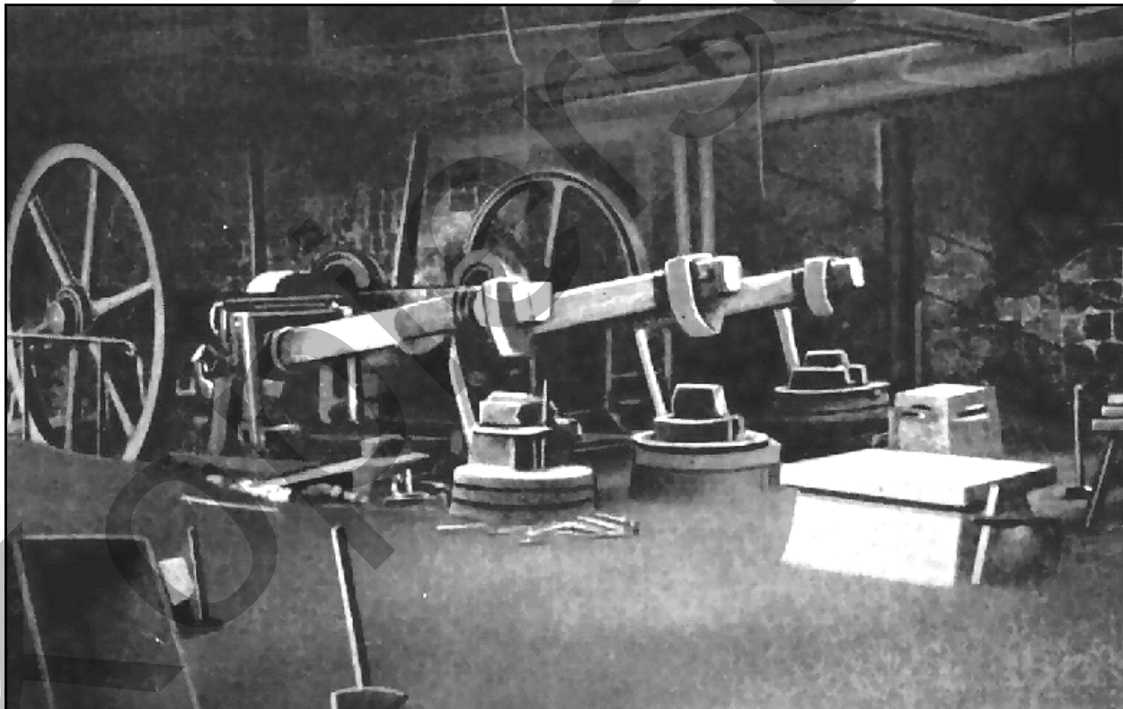
Abb. 5.13.4: Die drei Hämmer des Oberhammers. Foto: Archiv Berggießhübel.
